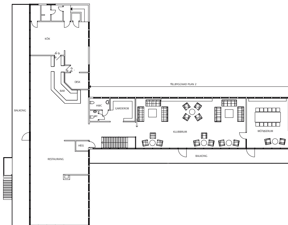
LJUNGHUSENS GOLFKLUBB UTREDNINGSSKISS TILLBYGGNAD PLAN 2
