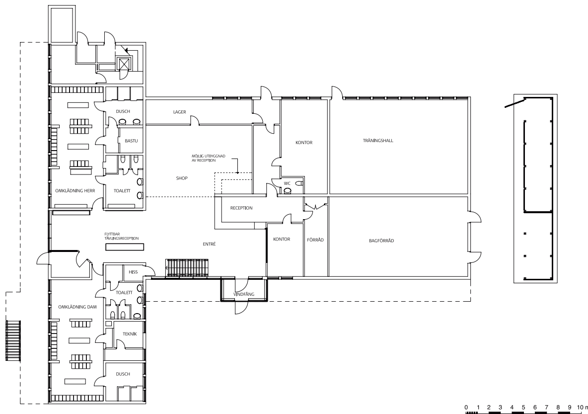
LJUNGHUSENS GOLFKLUBB UTREDNINGSSKISS BOTTENPLAN
